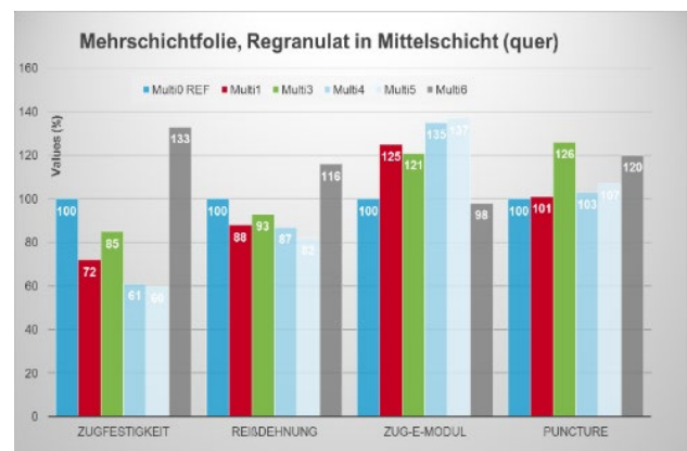
Abb. 13b: Mechanik regranulathaltiger Mehrschichtfolien (quer)
